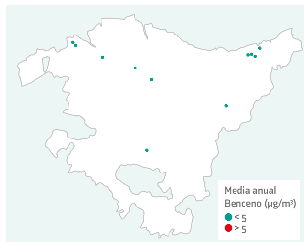
FIGURA 39. VALOR LÍMITE ANUAL DE BENCENO PARA EL AÑO 2021
