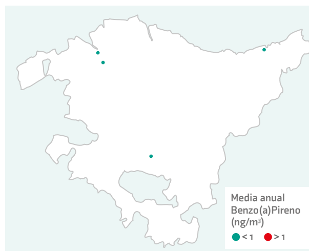
FIGURA 45. VALOR OBJETIVO DE BENZO(A)PIRENO PARA EL AÑO 2021
