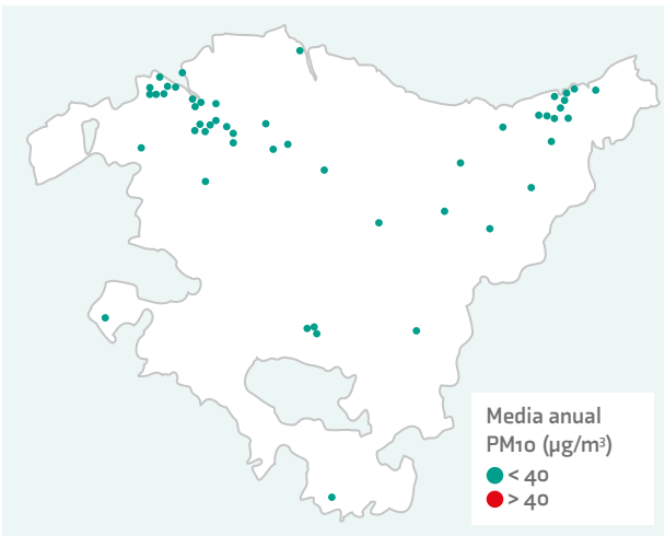
FIGURA 27. CUMPLIMIENTO DEL VALOR LÍMITE ANUAL PARA LAS PARTÍCULAS PM 10 PARA EL AÑO 2021
