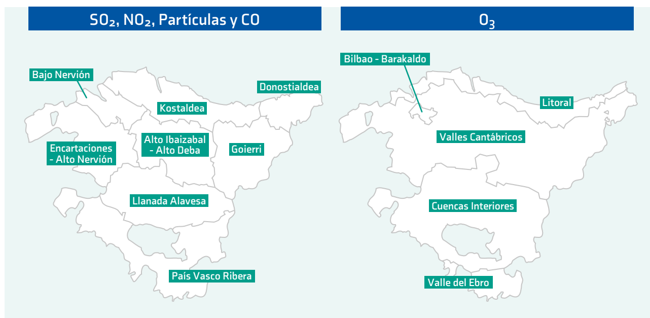
FIGURA 22. ZONIFICACIÓN DE EUSKADI PARA LA EVALUACIÓN DE LA CALIDAD DE AIRE
