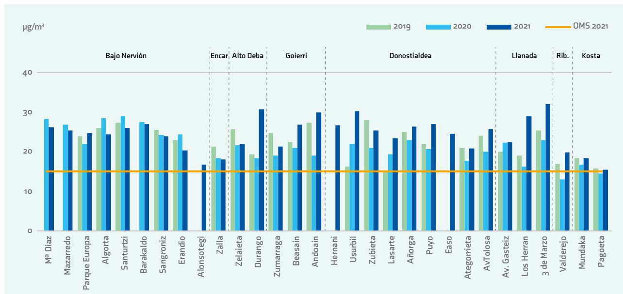
FIGURA 62. PERCENTIL 99 DE LOS VALORES MEDIOS DIARIOS DE PM 2,5 EN LOS ÚLTIMOS 3 AÑOS
