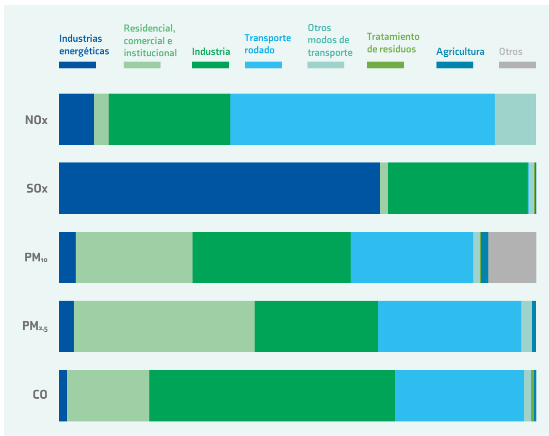
FIGURA 3. CONTRIBUCIÓN DE LOS DIFERENTES SECTORES AL TOTAL DE EMISIONES DE CADA CONTAMINANTE (AÑO 2019 11 )
