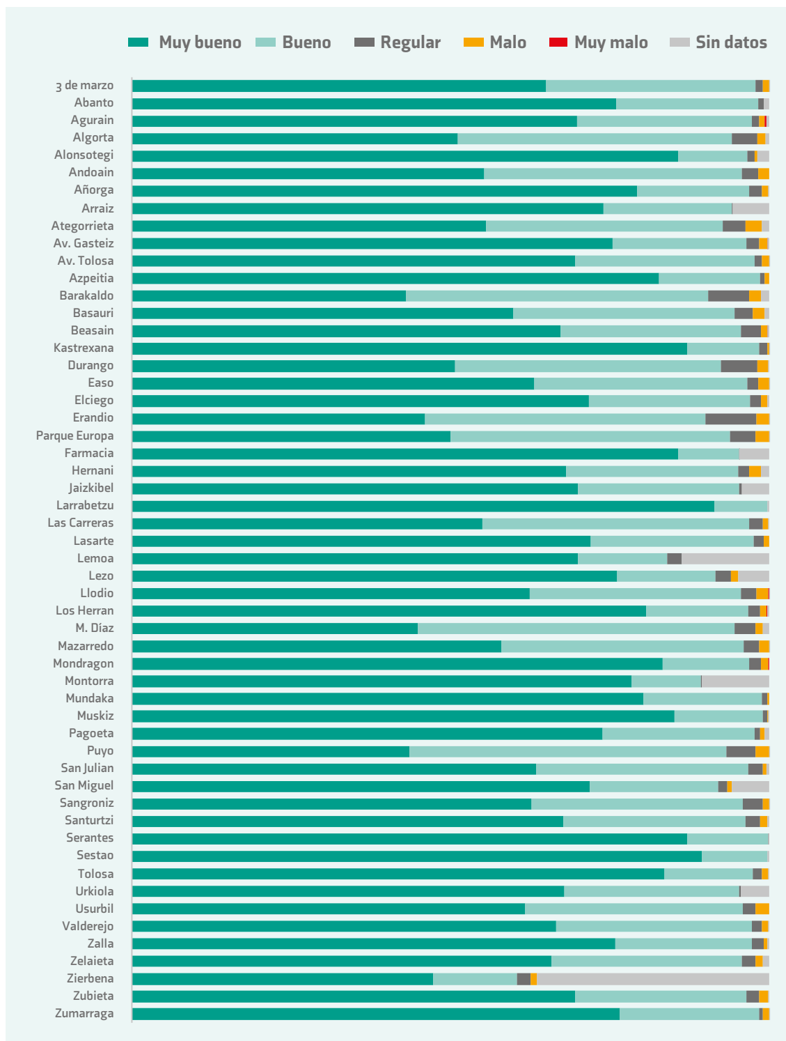
FIGURA 5. N° DE HORAS CON CADA TIPO DE ÍNDICE DE CALIDAD DEL AIRE EN LAS ESTACIONES PARA EL AÑO 2021
