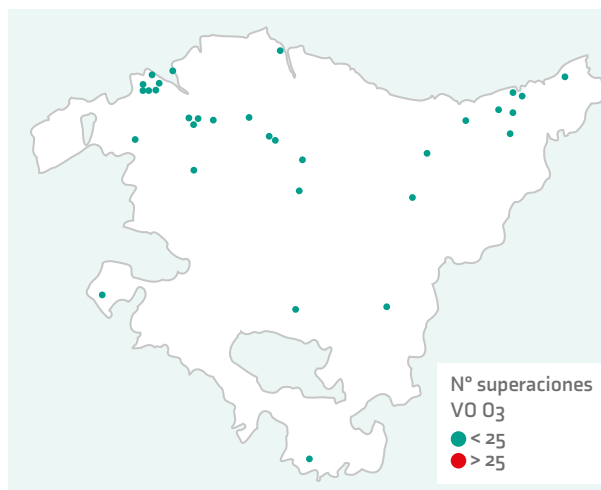
FIGURA 41. VALOR OBJETIVO PARA LAS OCTO HORARIAS MÓVILES DE O 3 PARA EL AÑO 2021
