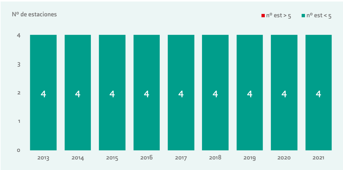
FIGURA 52. EVOLUCIÓN DE LAS ESTACIONES RESPECTO AL VALOR OBJETIVO DE CADMIO (2013-2021)
