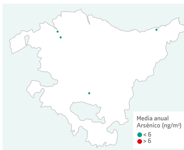
FIGURA 49. VALOR OBJETIVO DE ARSÉNICO PARA EL AÑO 2021
