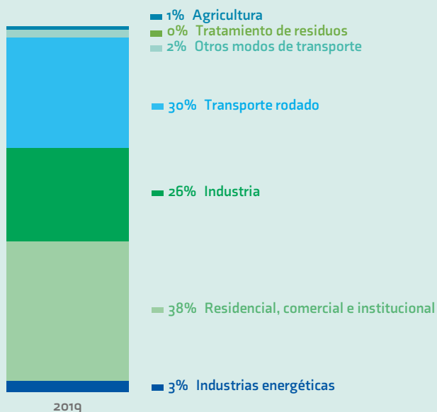
FIGURA 12. DISTRIBUCIÓN DE LAS EMISIONES DE PARTÍCULAS PM 2,5 POR SECTOR DE ACTIVIDAD
