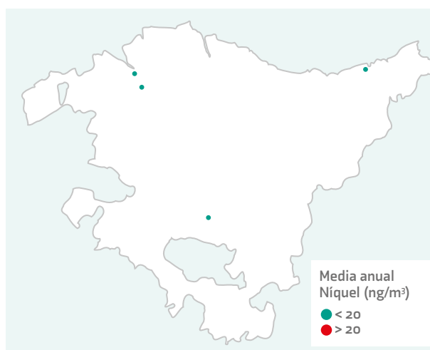
FIGURA 53. VALOR OBJETIVO DE NÍQUEL PARA EL AÑO 2021
