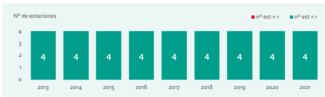
FIGURA 46. EVOLUCIÓN DE LAS ESTACIONES RESPECTO AL VO DE BENZO(A)PIRENO (2013-2021)
