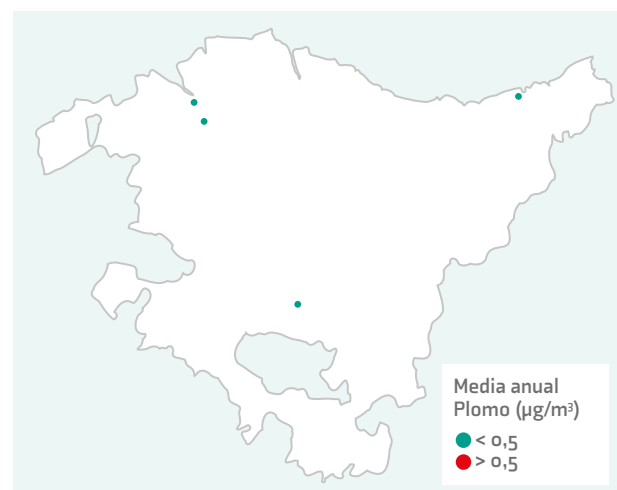
FIGURA 47. VALOR LÍMITE ANUAL DE PLOMO PARA EL AÑO 2021
