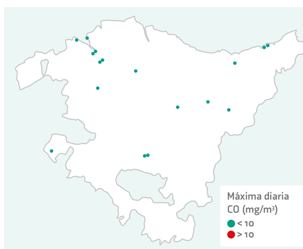
FIGURA 37. MÁXIMO OCTOHORARIO DE CO PARA EL AÑO 2021
