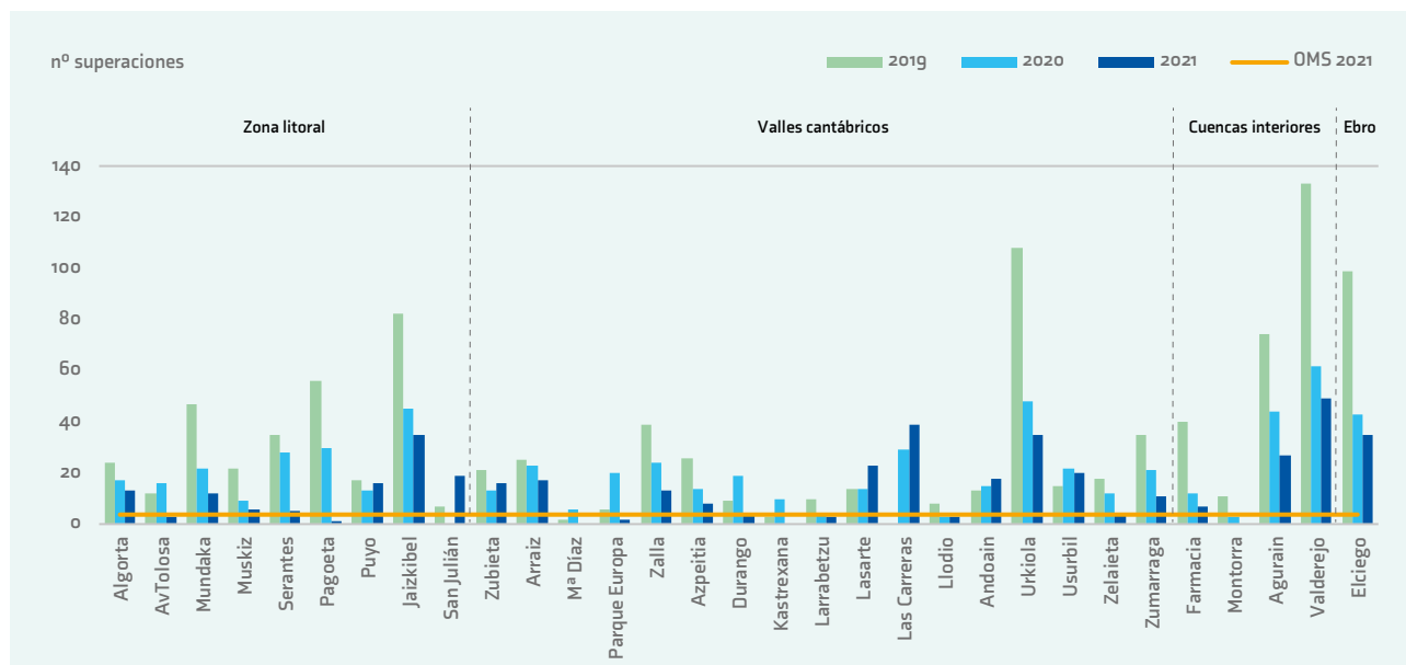
FIGURA 63. EVOLUCIÓN DEL Nº DE SUPERACIONES DE VALOR OCTOHORARIO DE O 3 EN LOS ÚLTIMOS 3 AÑOS
